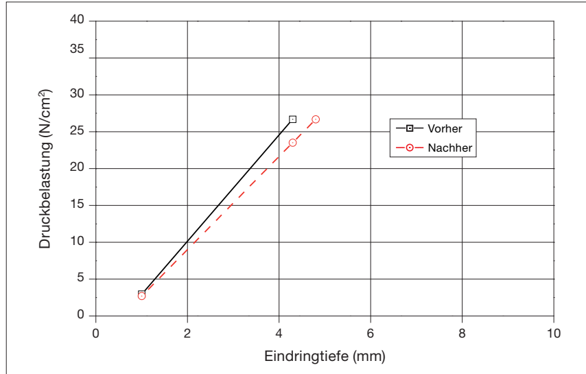
Bild 2: Verformbarkeit in Abhängigkeit vom Auflagedruck
