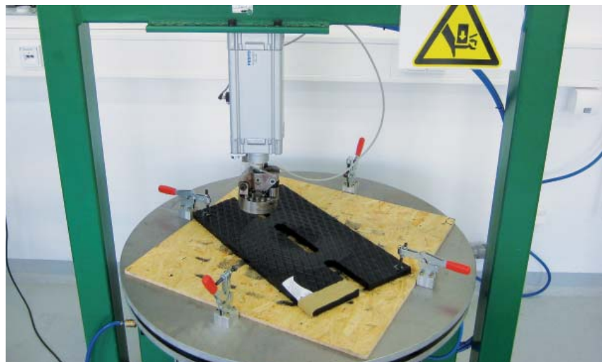
Bild 3: Prüfstand für Dauertrittbelastung
