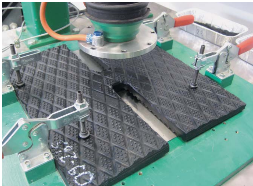
Bild 6: Testmuster nach dem Abriebtest
